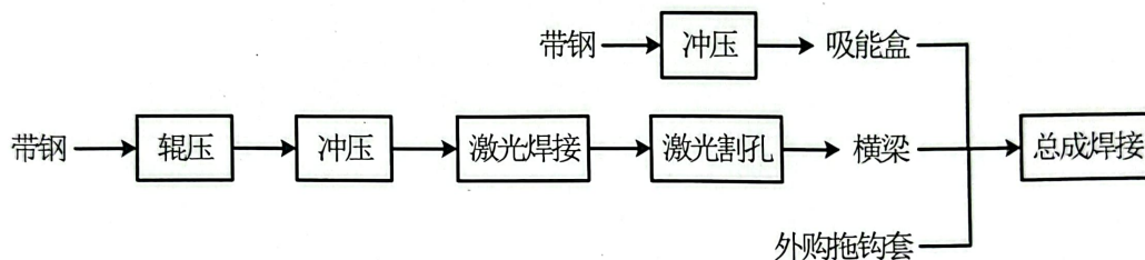
图2 保险杠生产工艺流程图
