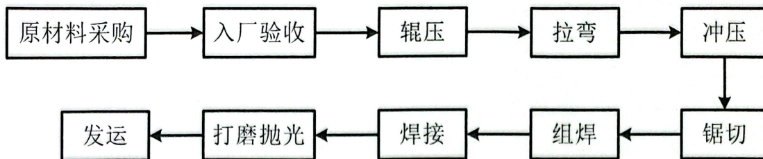
图1 车门框加工生产工艺流程图
